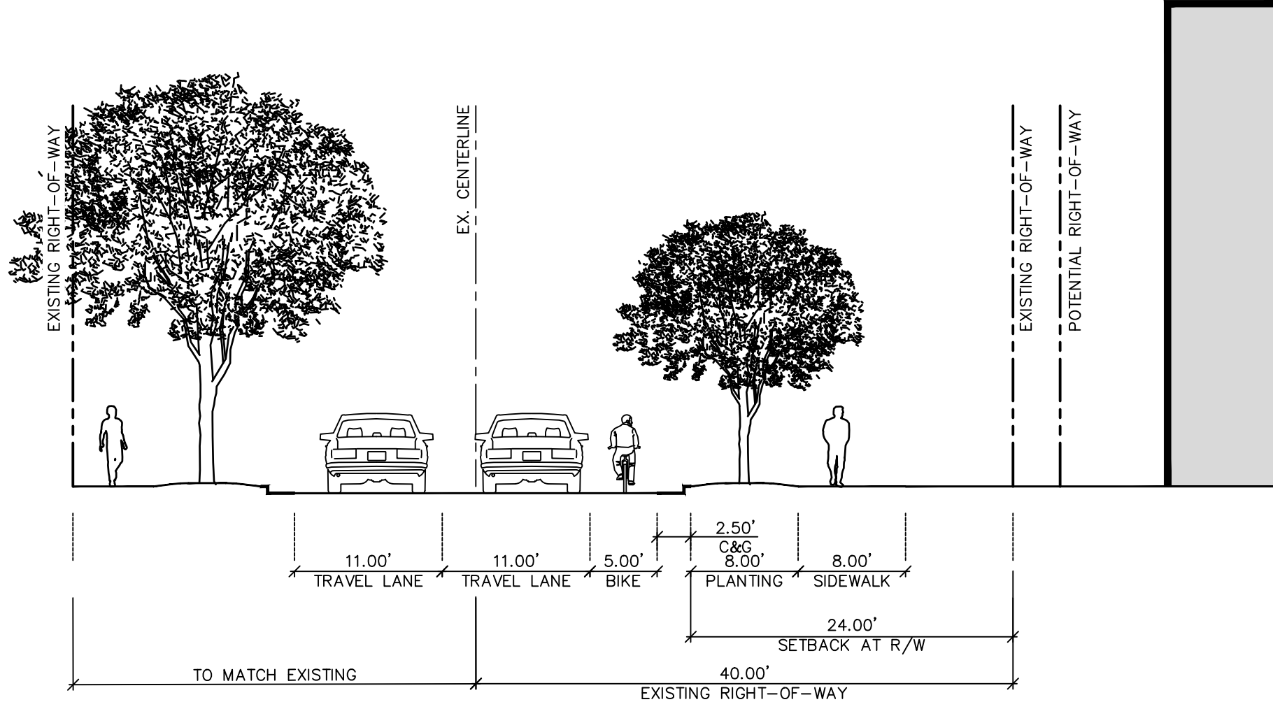
N. TRYON STREET CROSS SECTION SCALE: 1" = 10'-0"
